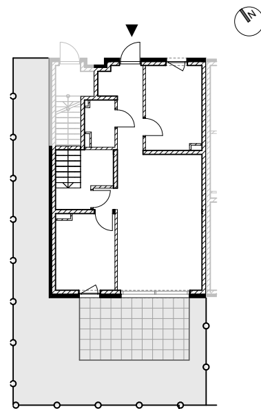
SCHEMAT DZIAŁKI
